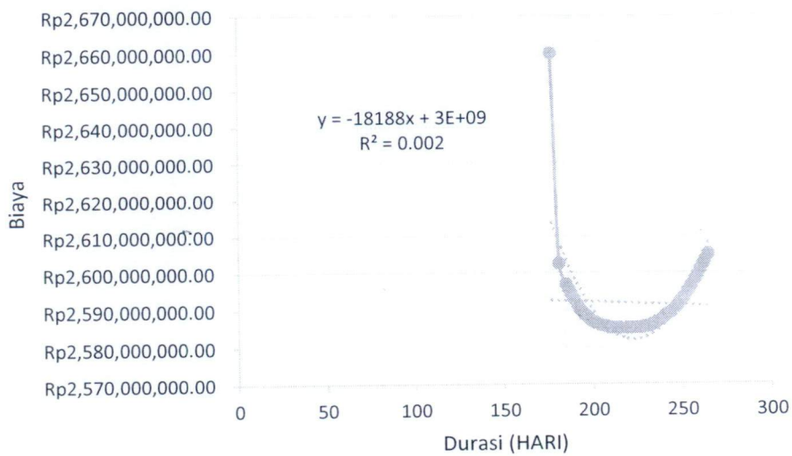
Gambar 5.10 Hubungan durasi dan biaya total akibat lembur 3 jam
