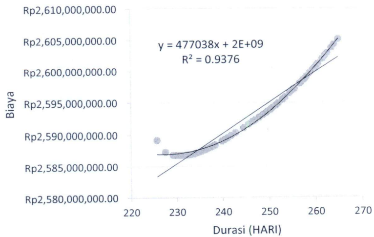
Gambar 5.4 Hubungan durasi dengan biaya total akibat lembur 1 jam
