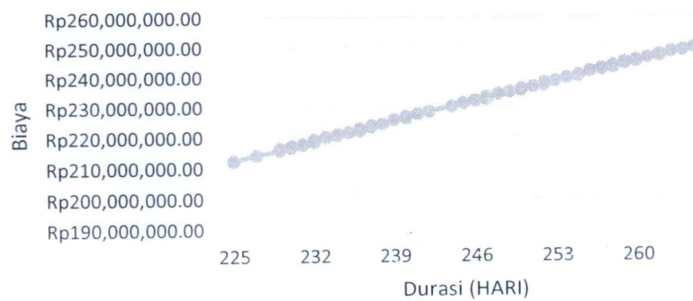
Gambar 5.2 Hubungan durasi dan biaya tidak langsung akibat lembur 1 jam
