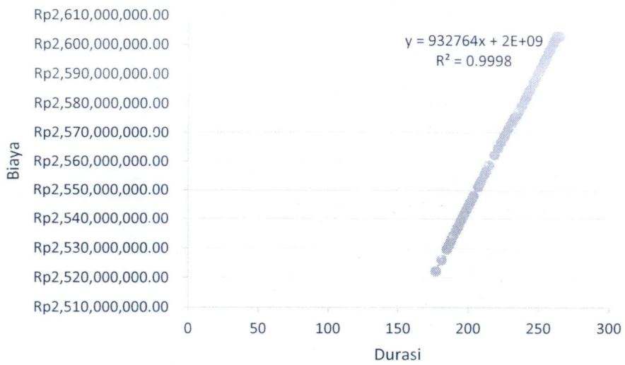
Gambar 5.20 Biaya total akibat penambahan tenaga kerja 3 jam
