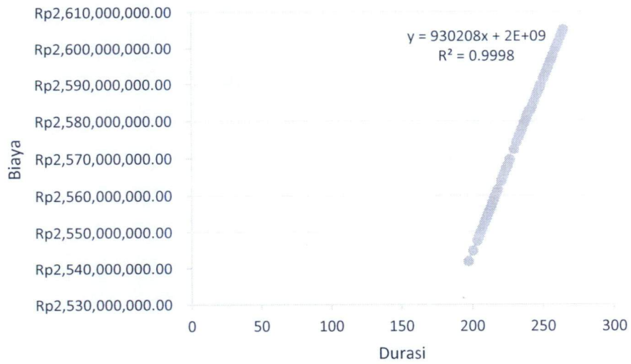
Gambar 5.17 Biaya total akibat penambahan tenaga kerja 2 jam
