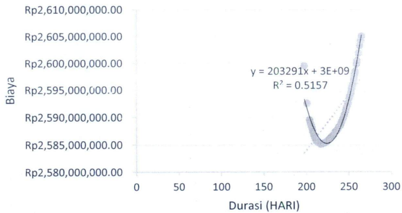
Gambar 5.7 Hubungan durasi dan biaya total akibat lembur 2 jam
