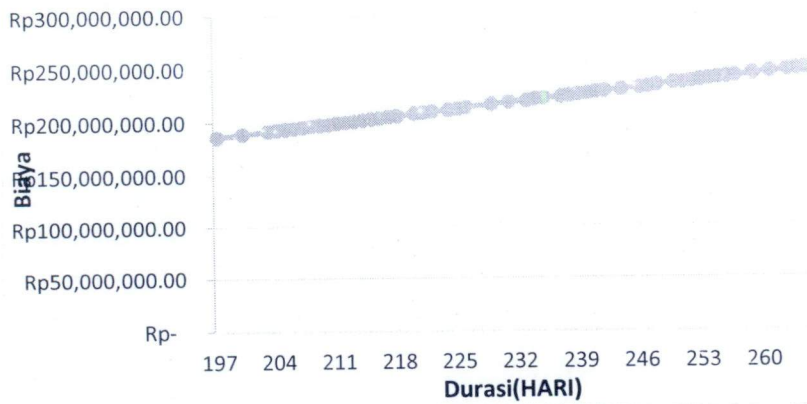
Gambar 5.5 Hubungan durasi dengan biaya tidak langsung akibat lembur 2 jam
